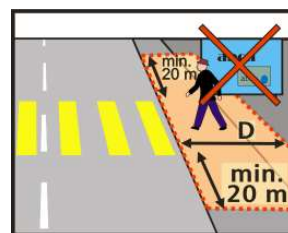
Verminderte Erkennbarkeit Fussgängerwarteraum (SSV Art. 96, Abs. 1, Bst. a)
