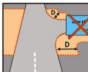
Sichtzonen bei Ausfahrten
