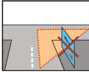
Sichtzonen der Verzweigungen (SN 640 273 / SSV Art. 96, Abs. 1, Bst. a)
